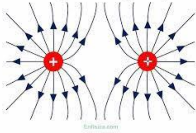
Líneas de campo eléctrico de dos cargas positivas iguales
