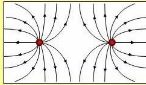
Líneas de campo eléctrico alrededor de dos cargas positivas.
