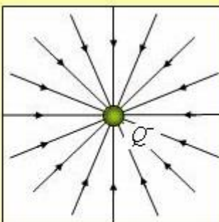
Líneas de campo eléctrico alrededor de una carga Q^- .
