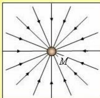
Líneas de campo gravitacional alrededor de una masa M .
